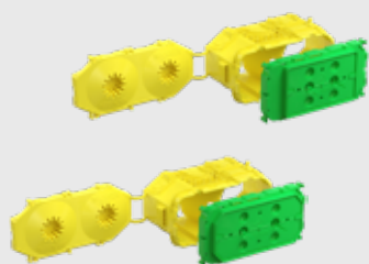
B1 Gerätedose für italienische Einbaugeräte, 3 Module / 4 Module 1269-03 | 1269-04
