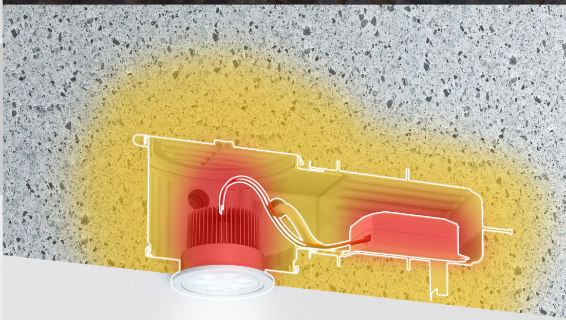
Stable, résistant aux charges élevées et facile à travailler. HaloX® permet un positionnement sûr de nouveaux éclairages ou haut-parleurs.
