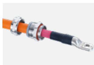
3. Dichteinsatz einschieben
