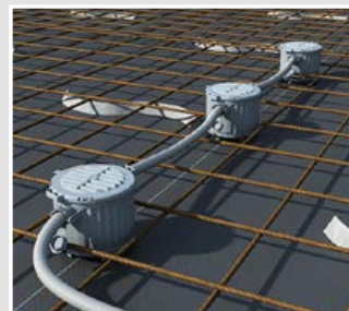
Groepsschakeling HS-halogenarmaturen.
