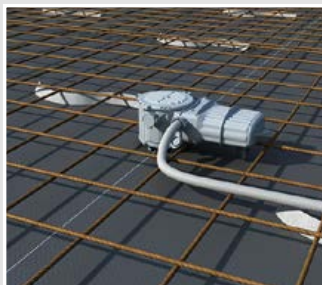
Aansluiting en buisvoer ledarmaturen met driver.
