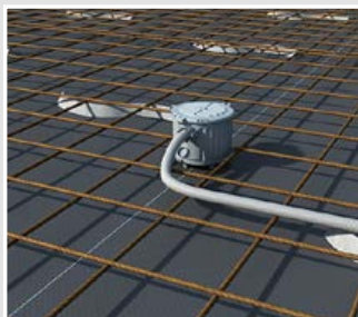
Aansluiting en buisvoer bij een 230V-ledarmatuur.
