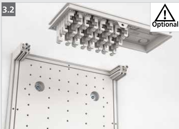
Modul in Gehäuseunterteil einfügen.
