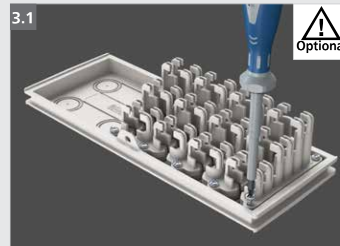
Optional: Zugentlastung auf Modul anschrauben.
