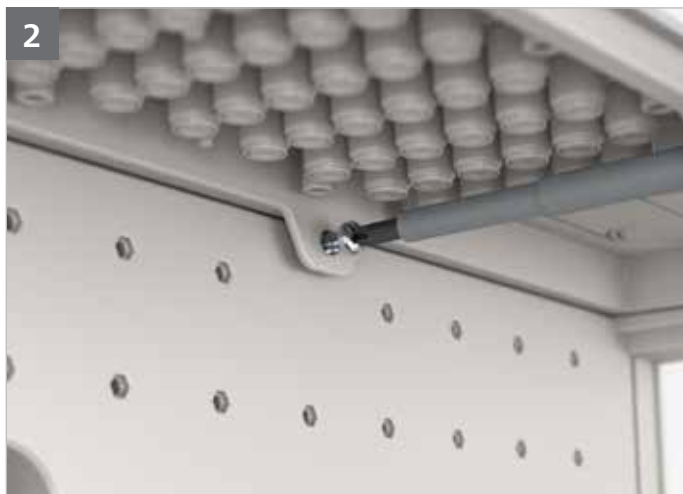
Wandmodul mittels Schraube im Gehäuse Unterteil fixieren. Hinweis: Sämtliche Wandmodule müssen mittels mitgelieferter Schrauben fixiert werden.
