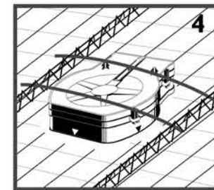
Gehäuse gegen Aufschwimmen durch Einschieben von Stahlstäben unter die Gitterträger sichern oder durch Befestigung des Rückteils mit Rödeldraht oder Kabelbindern an der Bewehrung.
