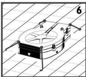
Gehäuse gegen Aufschwimmen durch Befestigung des Rückteils mit Rödeldraht oder Kabelbinder an der Bewehrung sichern. Anschließend betonieren.
