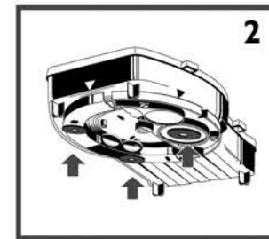
Nach Markieren der Position auf dem Schaltisch Frontteil über Markierungshilfen mit min. 4 Klebefolien (1219-00) anbringen ...
