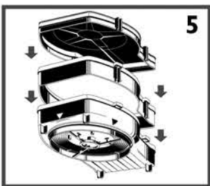
Rückteil (Evtl. Zwischenrahmen) auf Frontteil einrasten.
