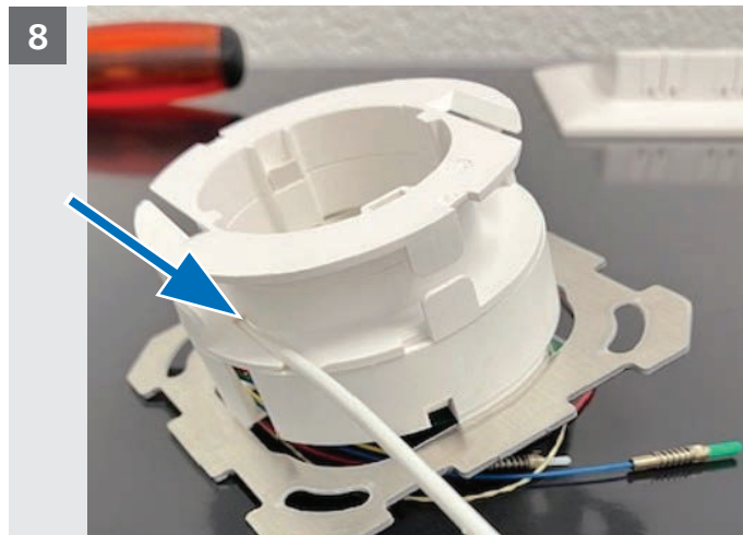
OTO UP Rondelle aufsetzen, Kabel durch Öffnung ziehen.
