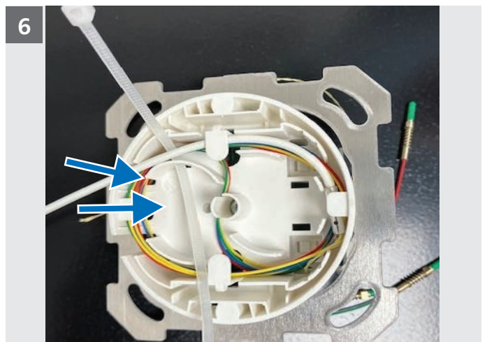
Fasereinführung OTO UP (4 Faser: Rot, Grün, Gelb, Blau). Ablegen der Fasern.
