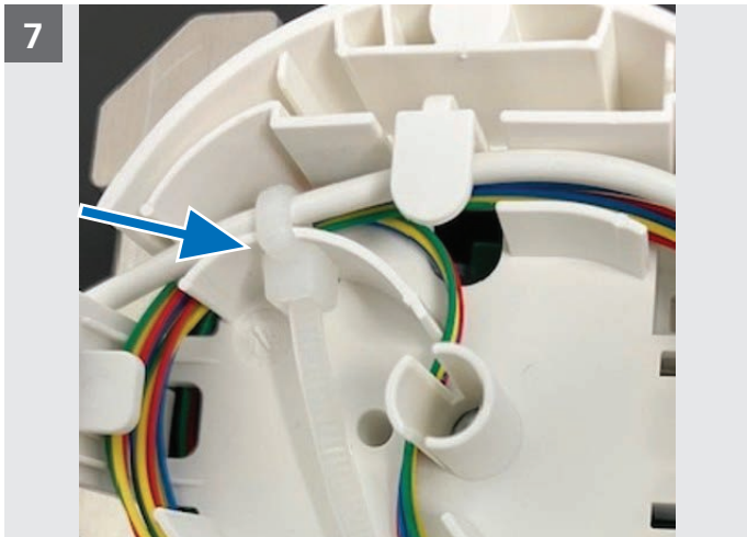
Fixierung mit Kabelbinder.
