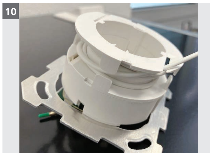
OTO UP Überlänge (Kabelreserve) auf die Rondelle aufrollen. Dose wieder zusammenstellen (Abdeckrahmen & Abdeckung).
