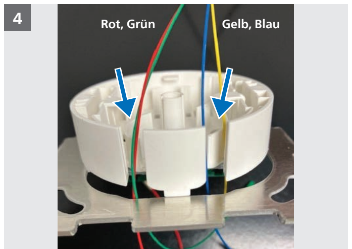
Kabeleinführung OTO UP (4 Faser: Rot, Grün, Gelb, Blau) / in Kupplung hinten einstecken.
