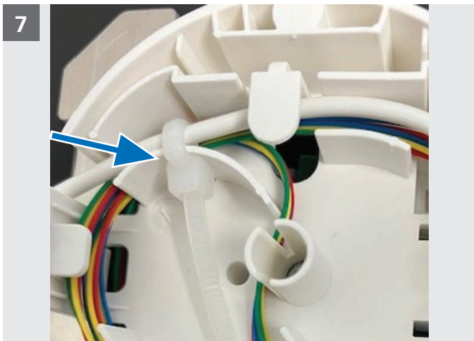
Fixation avec des colliers de serrage.
