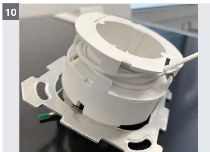
Avvolgere la lunghezza di cavo in eccesso (riserva) sul tondo. Rimontare il contenitore (telaio di copertura e coperchio).
