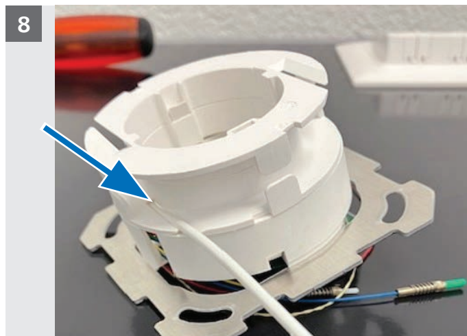
Posiziona il disco OTTO UP sulla base e fai passare il cavo attraverso l'apertura.
