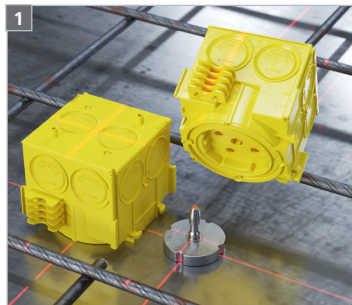
System-Haftmagnete (1299-69 / 1299-70). System magnet (1299-69 / 1299-70). Aimant de retenue du système (1299-69 / 1299-70). Systeem-hechtmagneet (1299-69 / 1299-70). Magneti di fissaggio del sistema (1299-69 / 1299-70).
