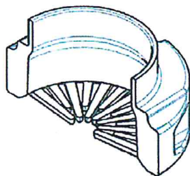
"Dichtdeckel", Halbschale
