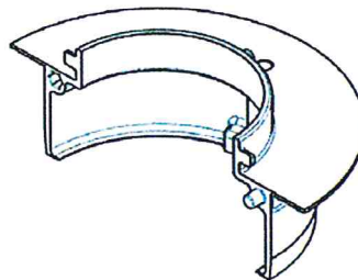
"Dichteinsatz", Halbzylinder
