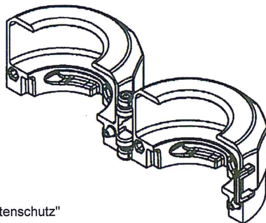
"Dichteinsatz", Halbzylinder
