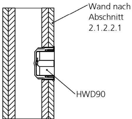
Einseitiger Einbau
