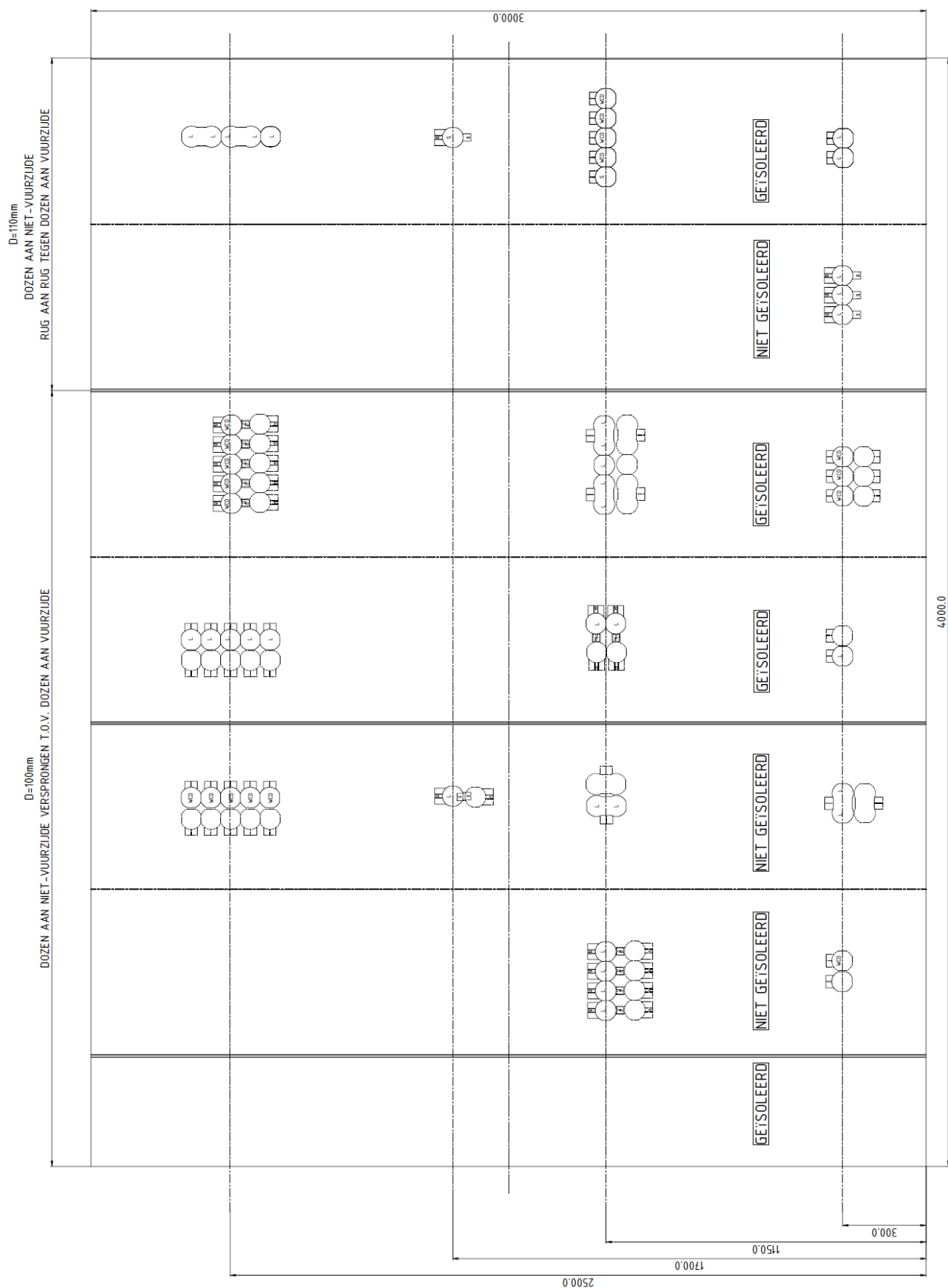
Figuur 2: Verhitte zijde van de wand voorzien van hollewandozen met verschillende typen bedrading
