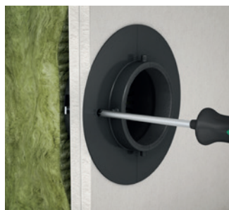
1 Vis FX4 | 2 Cylindre de cloisonnement | 3 Element d'étanchéité avec nervure de refroidissement
