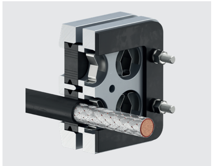
Querschnitt MCE EMV mit abgemantelterm Kabel
