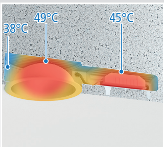
Temperaturprofil Einbaudownlight TC-TEL mit 2 x 26 W.
