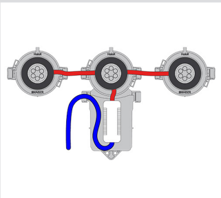
Schematische Darstellung Gruppenschaltung mit einem Betriebsgerät.
