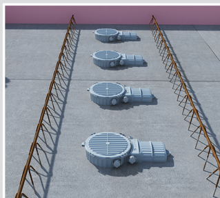
Erstelltes Fertigteillement mit integrierten HaloX-Gehäusen.
