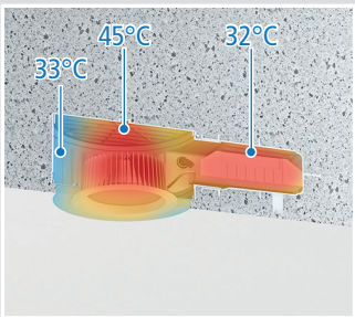
Temperaturprofil NV LED-Leuchte max. 35 W.
