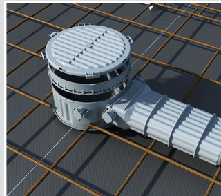
HaloX® 180: rückseitige Verlängerung 25 oder 50 (Art. Nr. 1282-25, -50).
