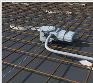
Anschluss und Rohreinführung LED-Leuchte mit Treiber.
