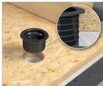
Befestigen des Wandanschlusselements durch die umlaufenden Dichtrippen in der Wandbeplankung.
