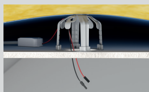
De afstandhouder staat stabiel op de beplating en verzekert de nodige afstand tot de isolatie.
